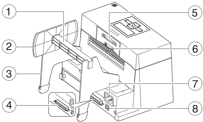
后视图
