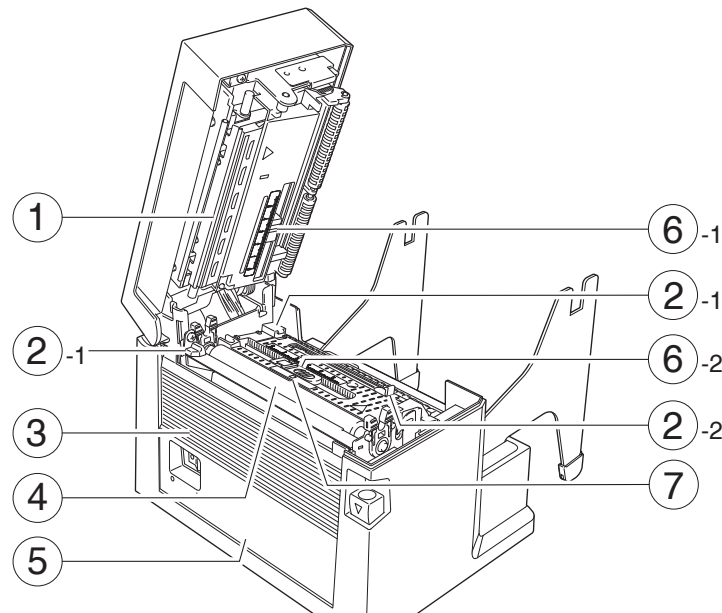
内视图
