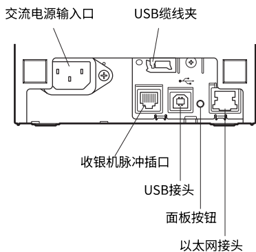
以太网 + USB
