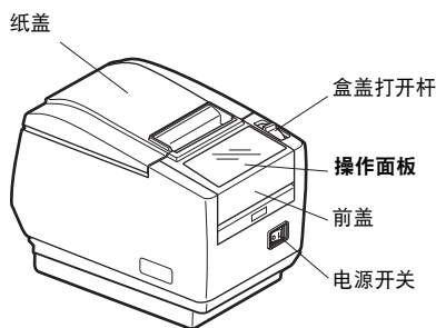
(正面图)
