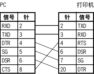
9 针 -25 针缆线
