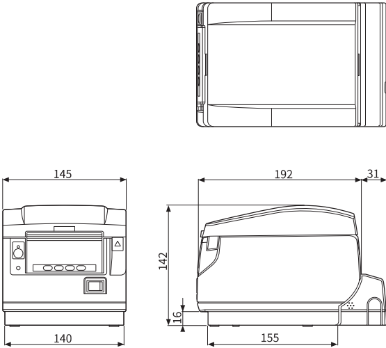
内置电源型
